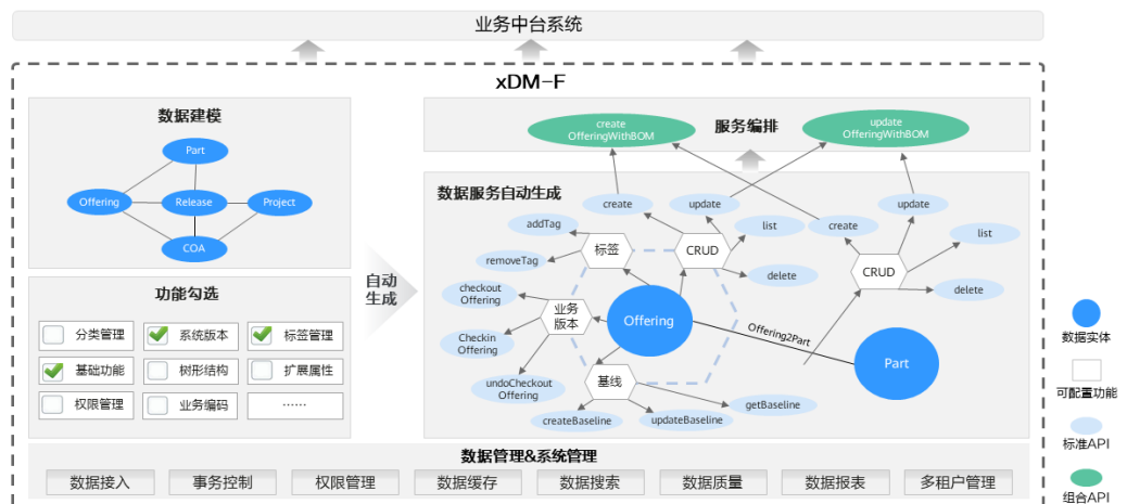
图 1-1 xDM-F 架构
